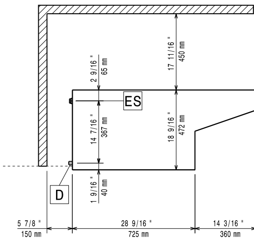
Zij aanzicht
